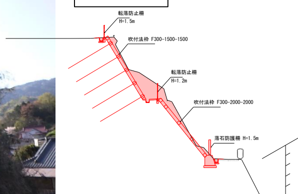
標準断面図
